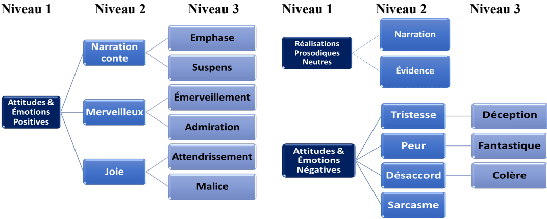
Figure 2 : Étiquettes sémantico-prosodiques
